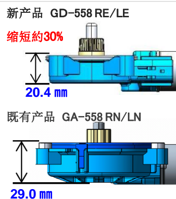
和既有产品的齿轮盒部位尺寸比较图
